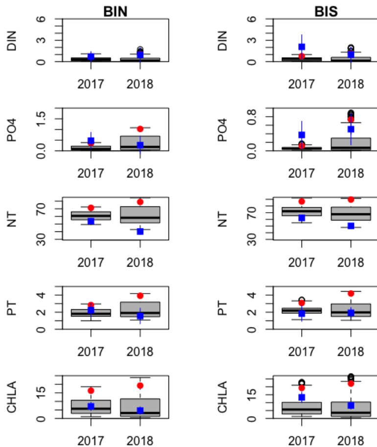
Figure 6. Variabilité (boxplot) des concentrations estivales simulées pour le NID, PID, NT, PT (µM) et Chl a (µg/l) dans les bassins nord (BIN) et sud (BIS) de la lagune de Biguglia en 2017 et 2018. Les percentiles 90 issus calculés à partir des sorties de modèle sont symbolisés par un cercle rouge, les moyennes estivale et écart-types des observations issues du RSL-DCE sont symbolisées par le carré bleu et segments bleus.
